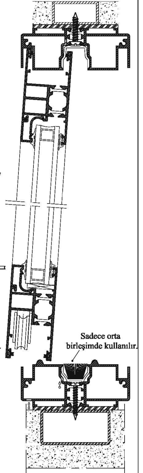
3.) KANAT SÖKÜLMESİ
