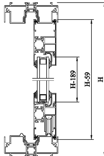
C-C Kesiti
