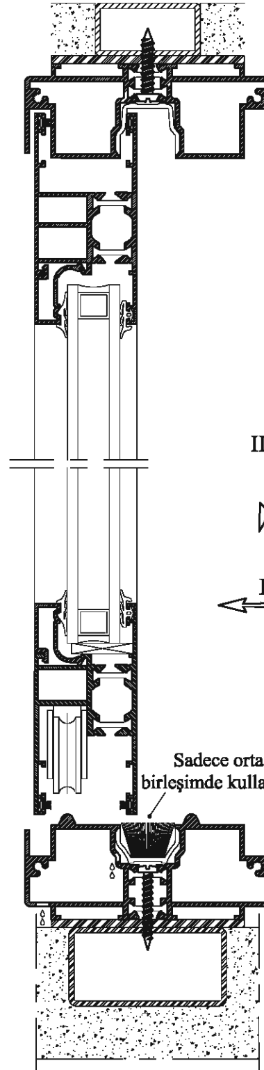
2.) KANAT SÖKÜLMESİ İÇİN KALDIRILMIŞ HALİ
